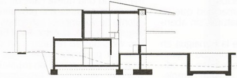
73 · SECCIÓN
