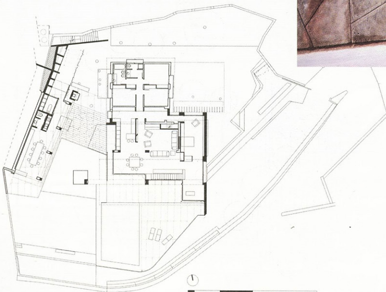
76 · PLANTA
