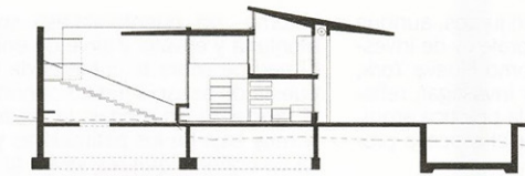
72 · SECCIÓN
